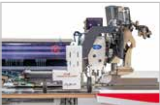
Step Motorla hassasiyeti artırılmış tela ünitesi Precision-enhanced interlining unit with stepper motor
